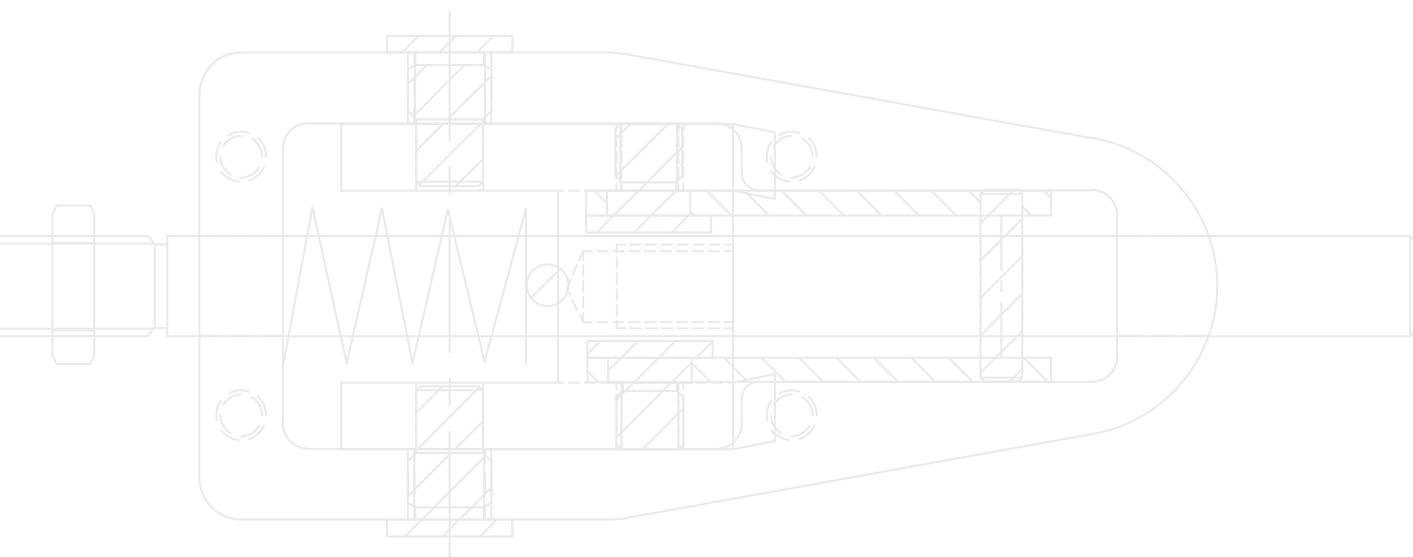
Mecanismo de presión accionado por muelle
